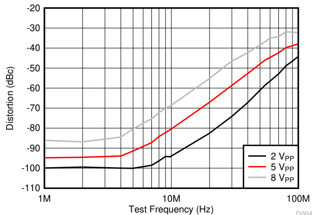
图 6-4. HD3 vs Frequency
