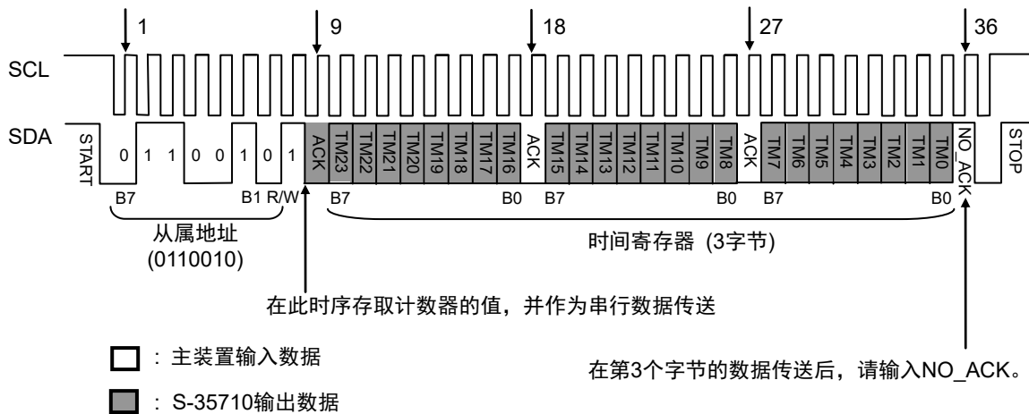
图27 时间寄存器的读出时序
