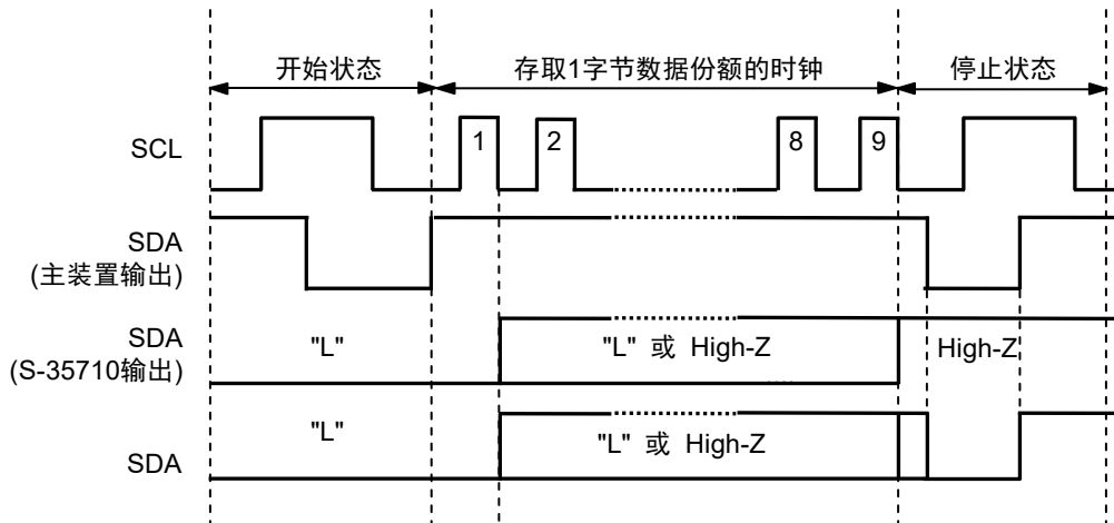
图30 SDA的释放方法
