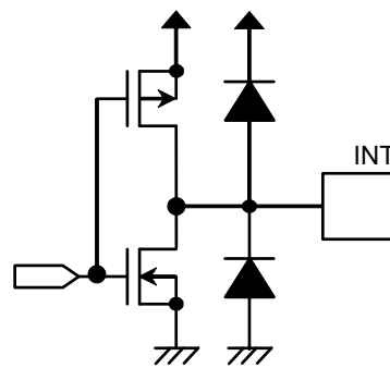
图8 INT端子 (CMOS输出)
