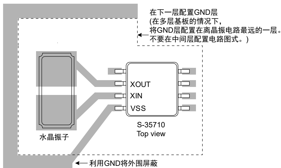
图38 连接布局图的推荐例
