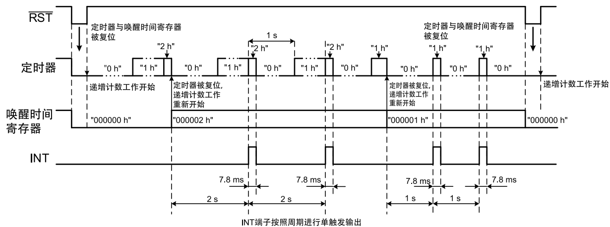
图13 单触发循环终止的输出时序例 (CMOS输出)
