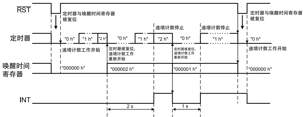
图19 握手协议终止的输出时序例 (CMOS输出)
