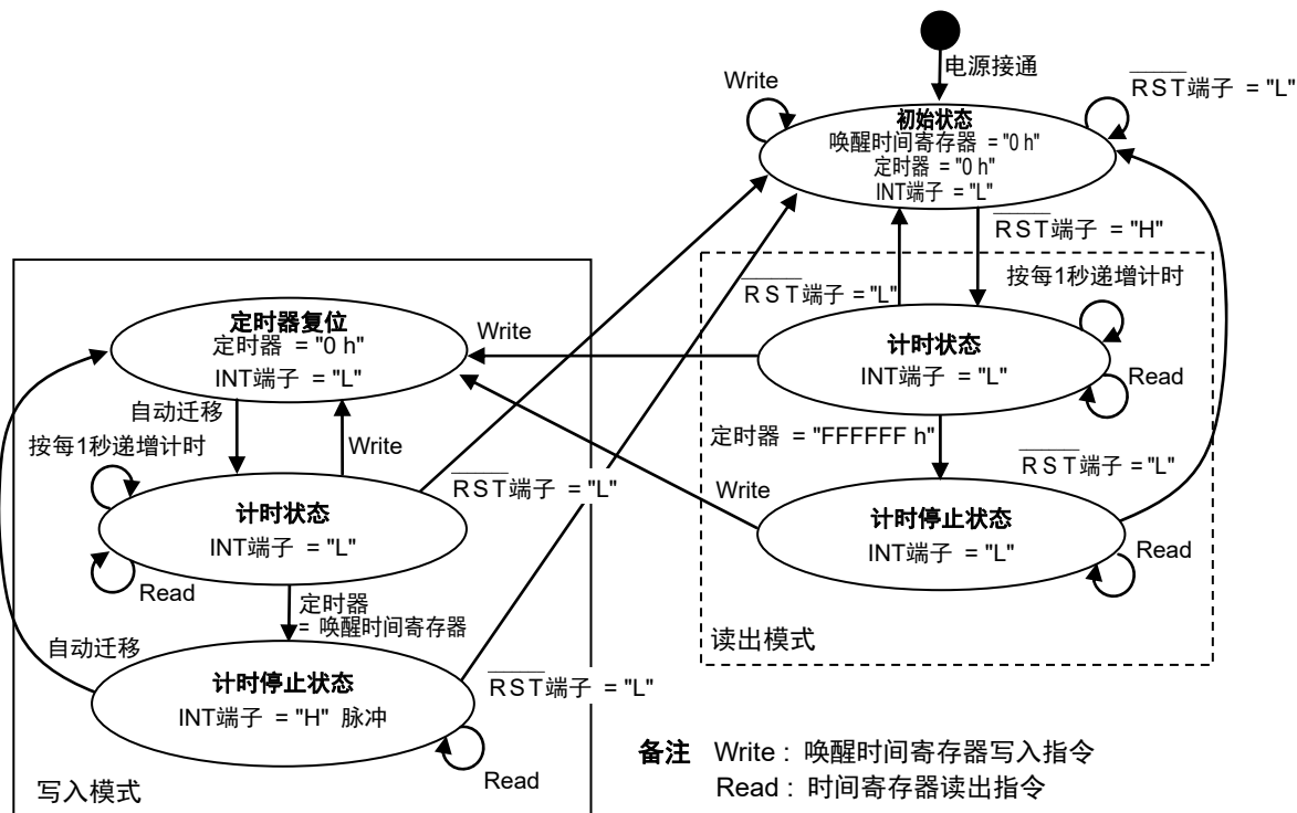
图17 单触发循环终止的状态迁移图 (CMOS输出)
