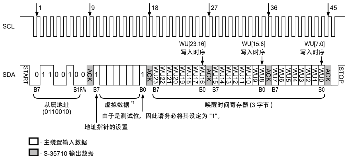
图28 唤醒时间寄存器的写入时序
