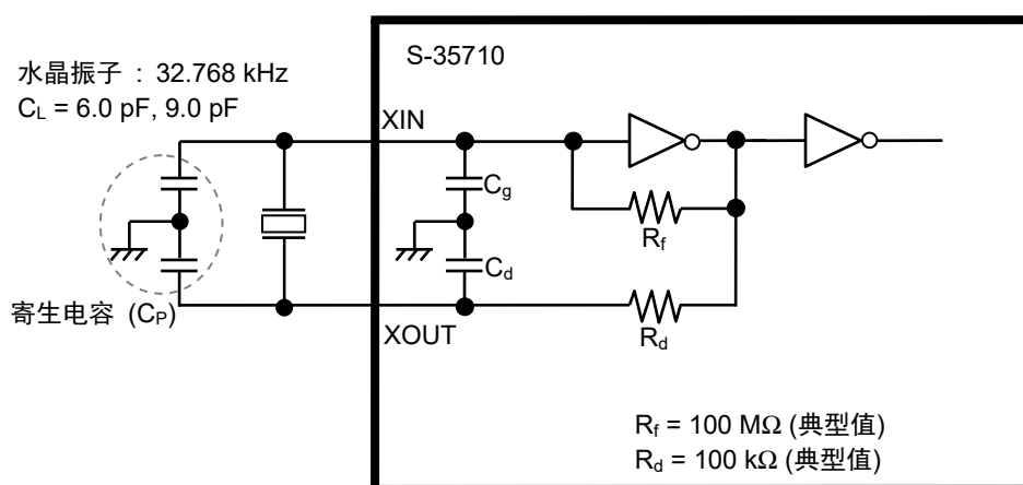
图37 晶振电路构成
