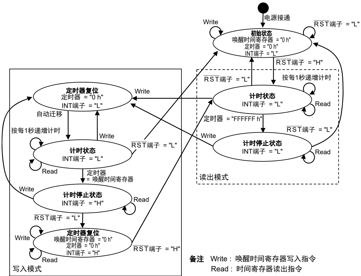
图21 握手协议终止的状态转移图 (CMOS输出)
