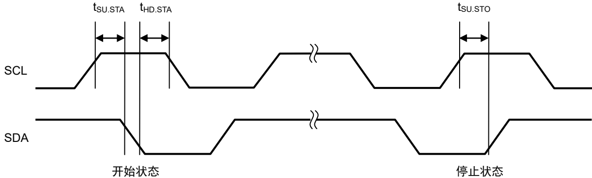
图24 开始 / 停止状态
