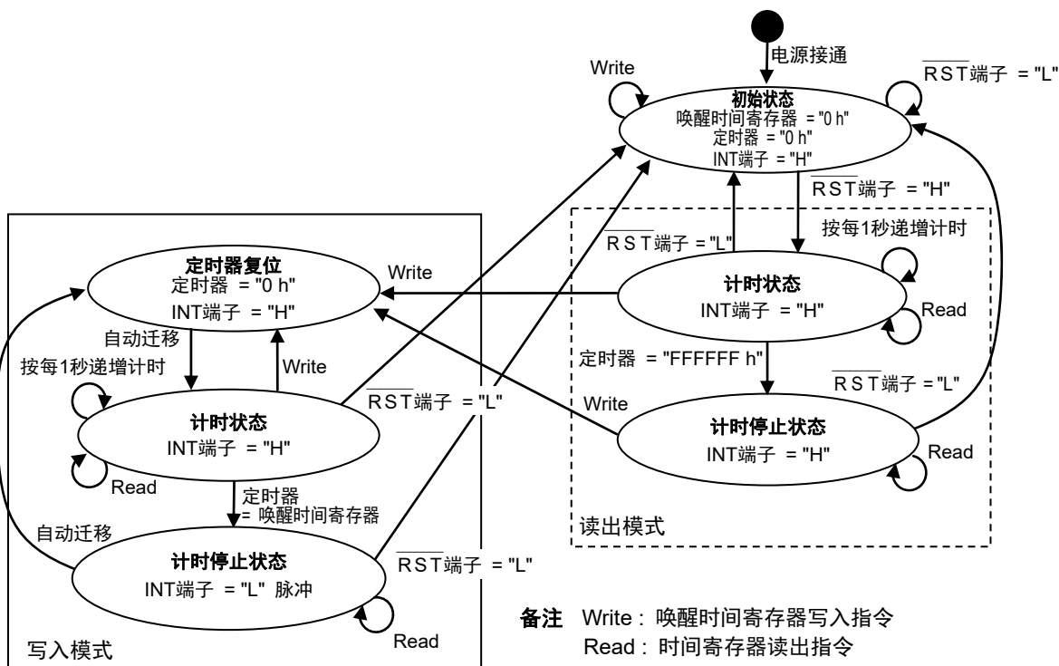
图16 单触发循环终止的状态迁移图 (N沟道开路漏极输出)
