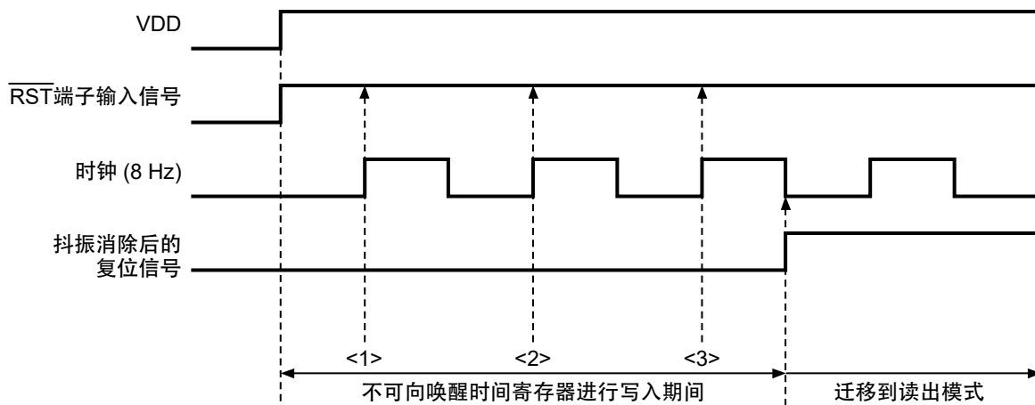
图35 电源接通时的时序图
