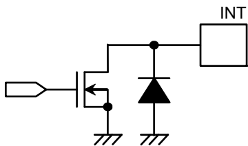
图7 INT端子 (N沟道开路漏极输出)
