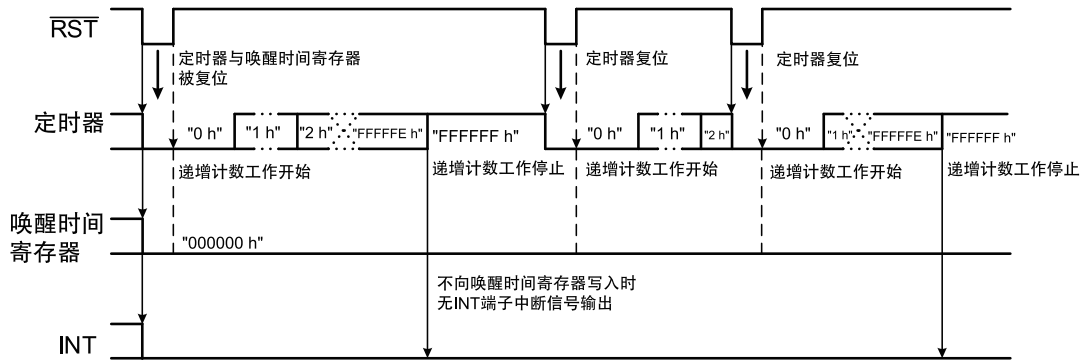
图14 不向唤醒时间寄存器写入时 (N沟道开路漏极输出)
