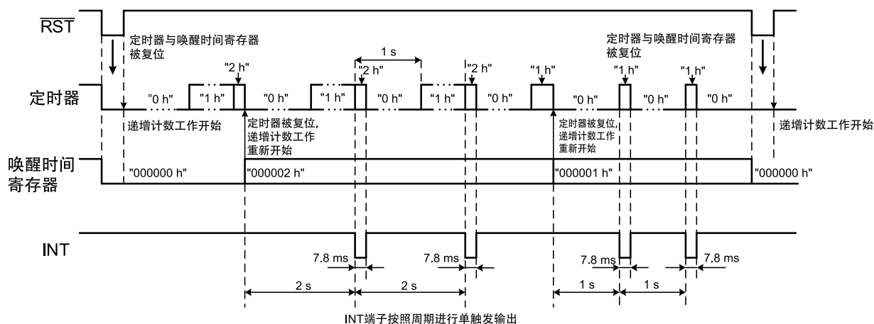
图12 单触发循环终止的输出时序例 (N沟道开路漏极输出)
