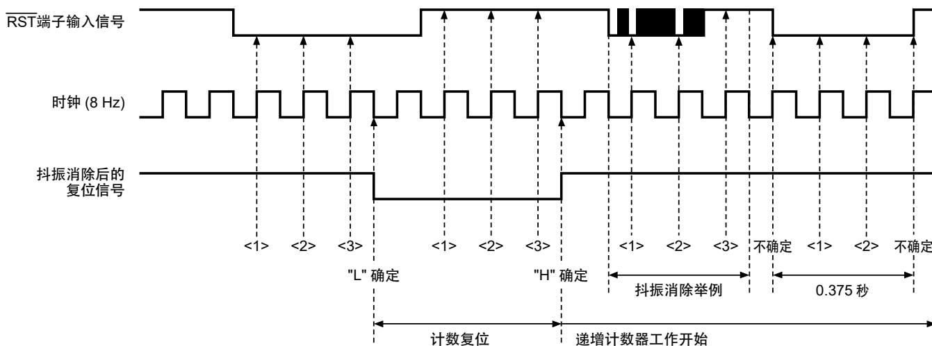
图34 抖振消除的时序图例
