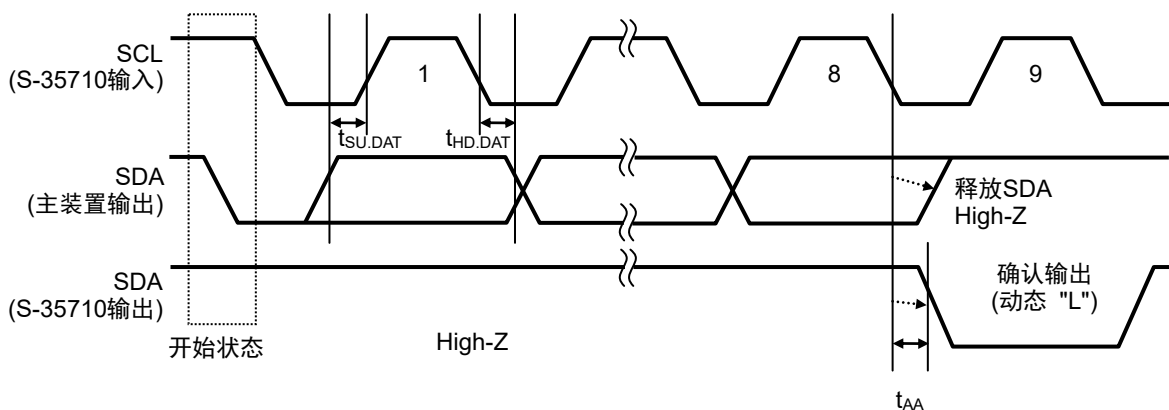
图25 确认输出时序
