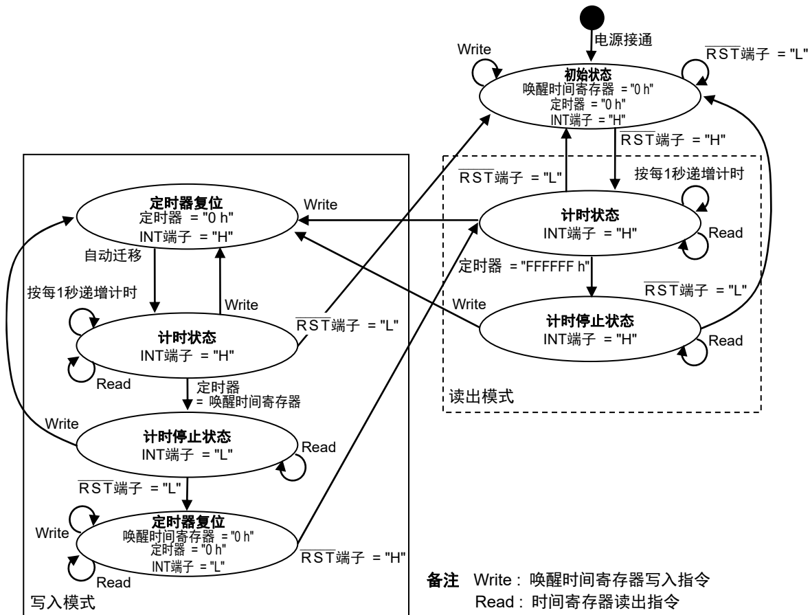
图20 握手协议终止的状态迁移图 (N沟道开路漏极输出)
