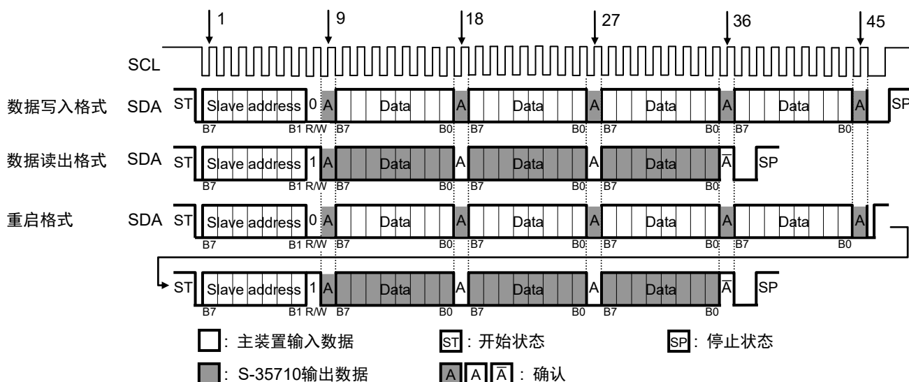
图26 串行接口的数据传送格式
