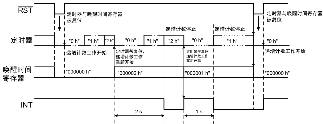
图18 握手协议终止的输出时序例 (N沟道开路漏极输出)
