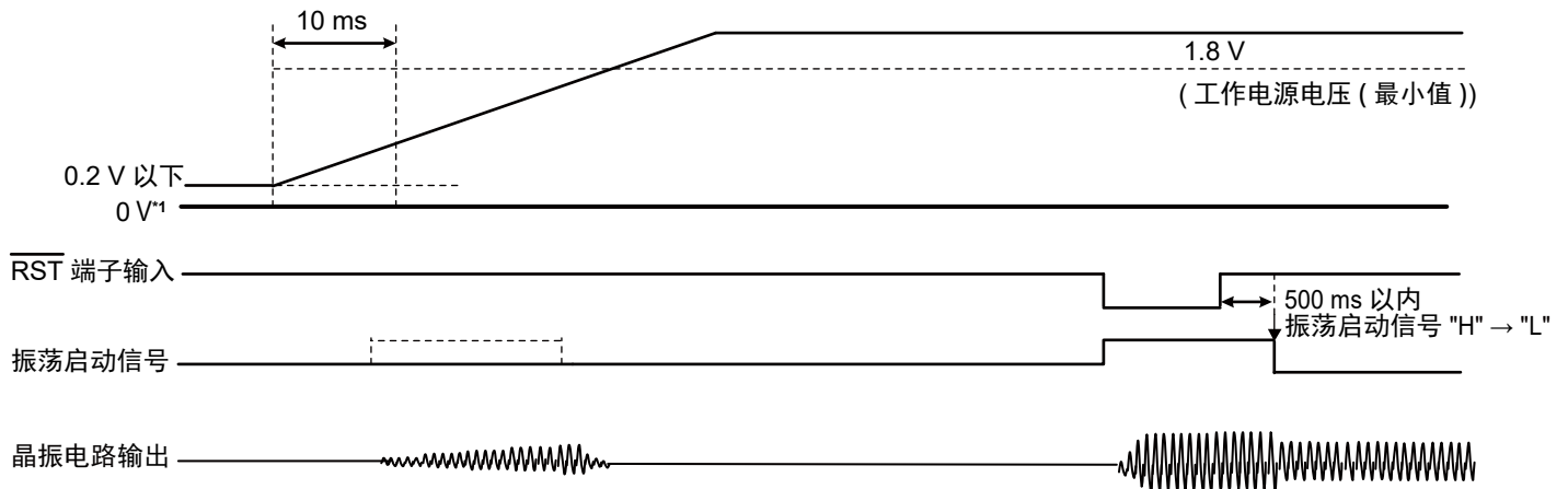
图33 \overline{\text{RST}} 端子 = "H" 时的电源电压上升
