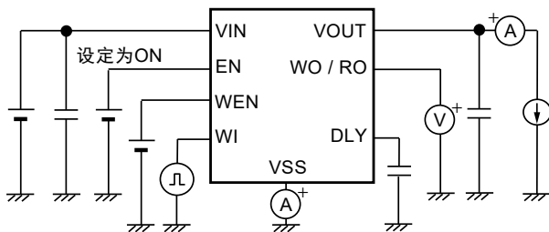
图17 测定电路9
