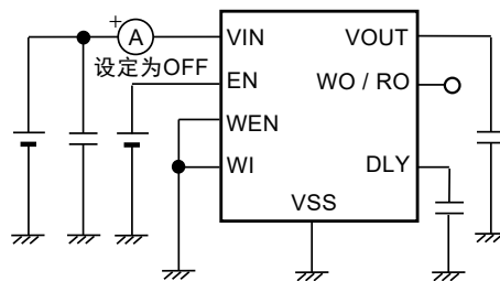
图18 测定电路10
