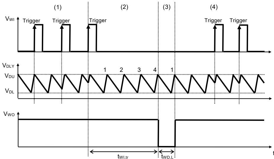
图35 看门狗定时器部分的时序图
