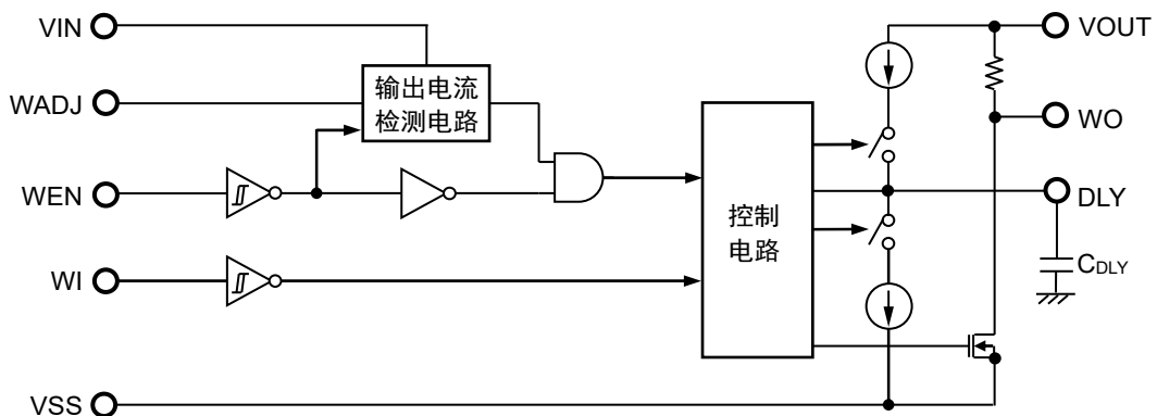
图36 看门狗定时器部分的工作说明图
