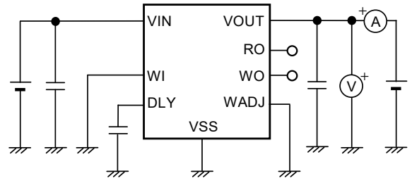
图21 测定电路2
