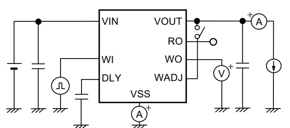
图29 测定电路10
