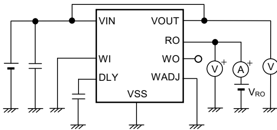
图24 测定电路5
