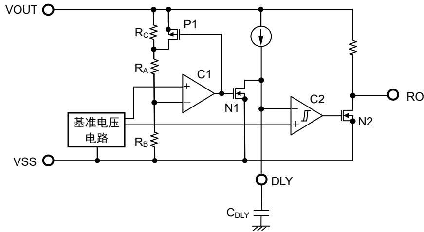
图33 检测器部分的工作说明图
