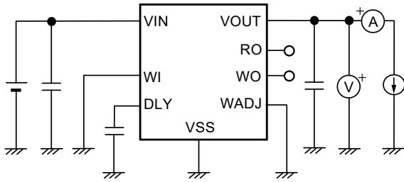
图19 测定电路1
