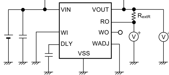
图22 测定电路4
