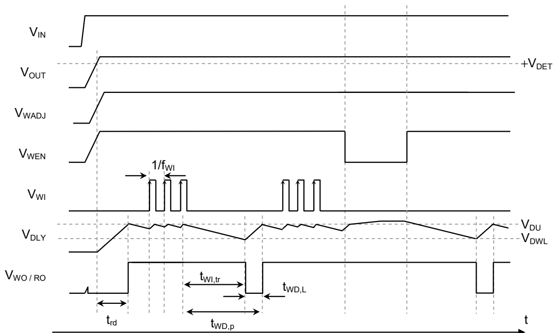
图40 看门狗定时器监视工作例2
