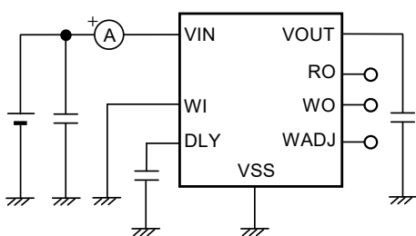
图27 测定电路9
