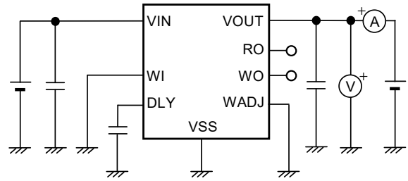
图20 测定电路2
