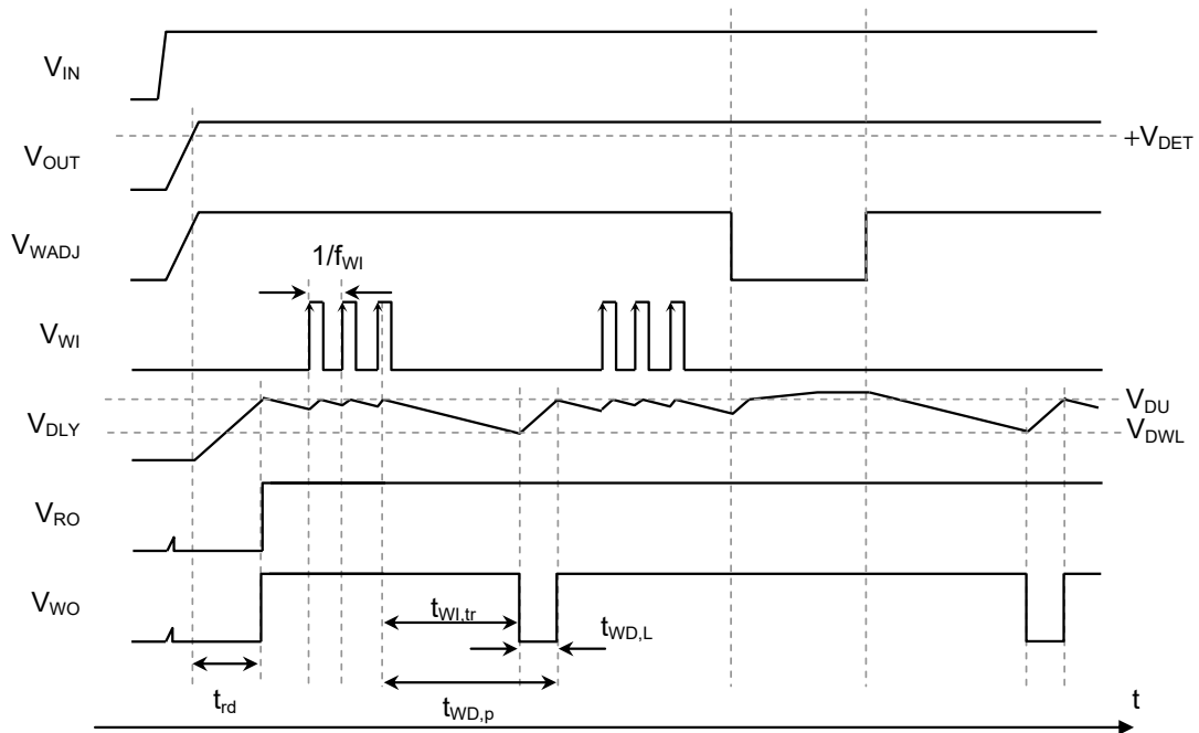
图42 看门狗定时器监视工作例
