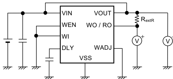
图12 测定电路4
