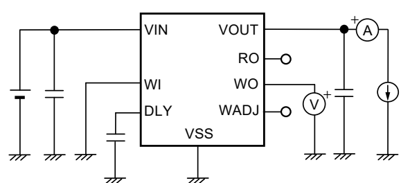
图24 测定电路6
