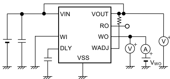
图29 测定电路11
