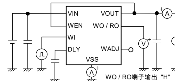
图17 测定电路9
