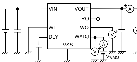
图25 测定电路7
