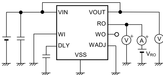
图23 测定电路5
