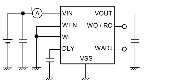
图18 测定电路10
