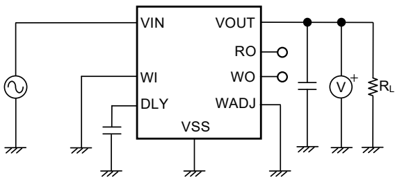
图21 测定电路3
