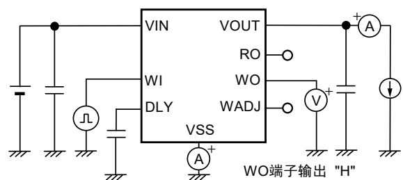
图26 测定电路8
