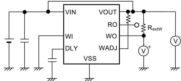
图28 测定电路10
