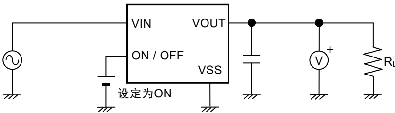
图7 测定电路5
