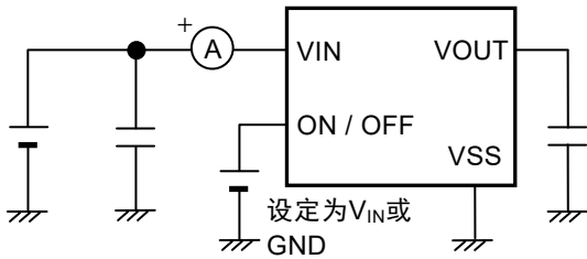
图4 测定电路2
