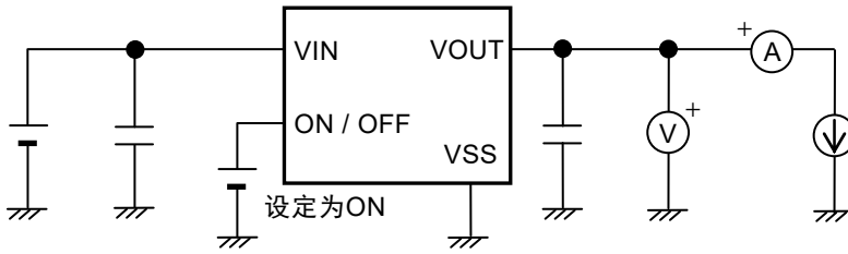
图3 测定电路1
