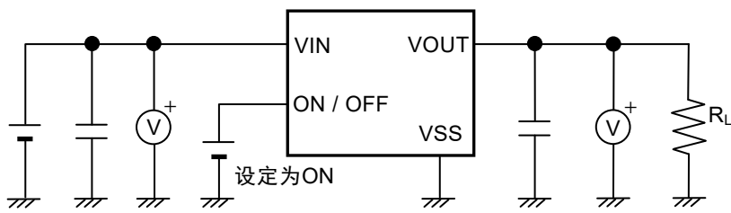
图13 抛负载特性的测定电路
