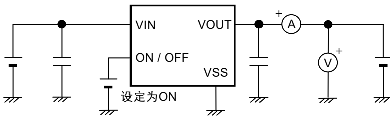
图5 测定电路3
