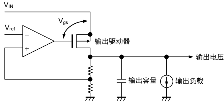
图11 电路图
