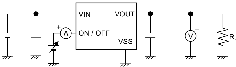
图6 测定电路4
