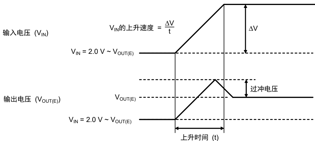
图12 V_{IN} 和过冲电压
