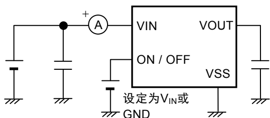
图5 测定电路2
