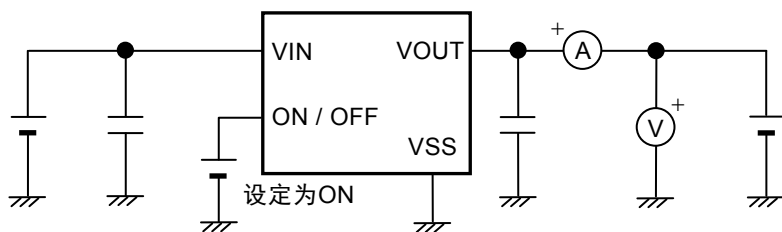
图6 测定电路3
