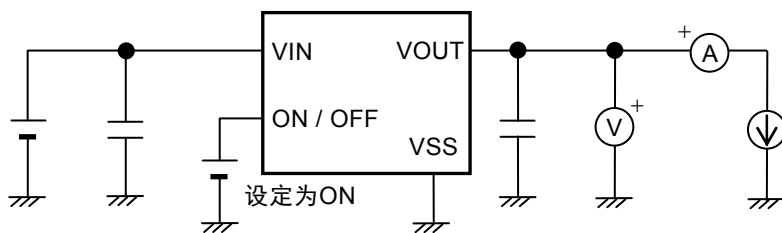
图4 测定电路1
