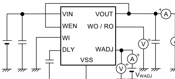
图18 测定电路7
