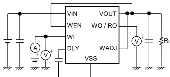
图19 测定电路8
