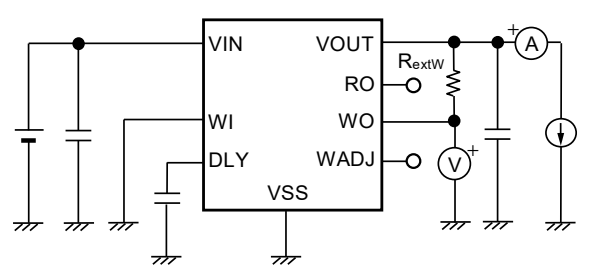
图27 测定电路6
