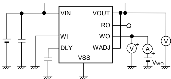
图30 测定电路9
